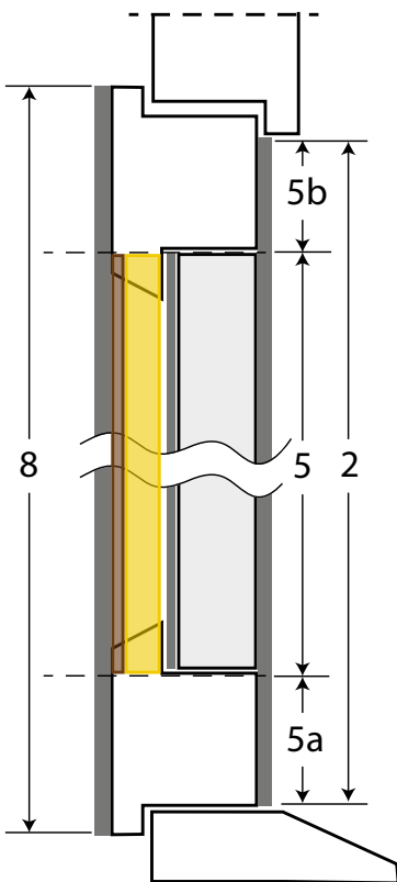
Coupe Verticale
