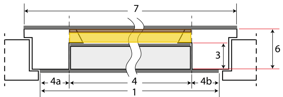
Coupe horizontale
