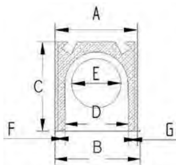
Sous-face PVC
